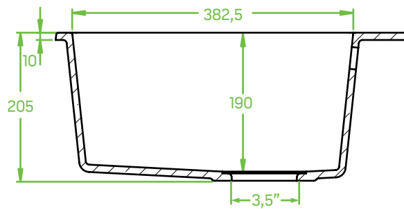
PRZEKRÓJ A-A
